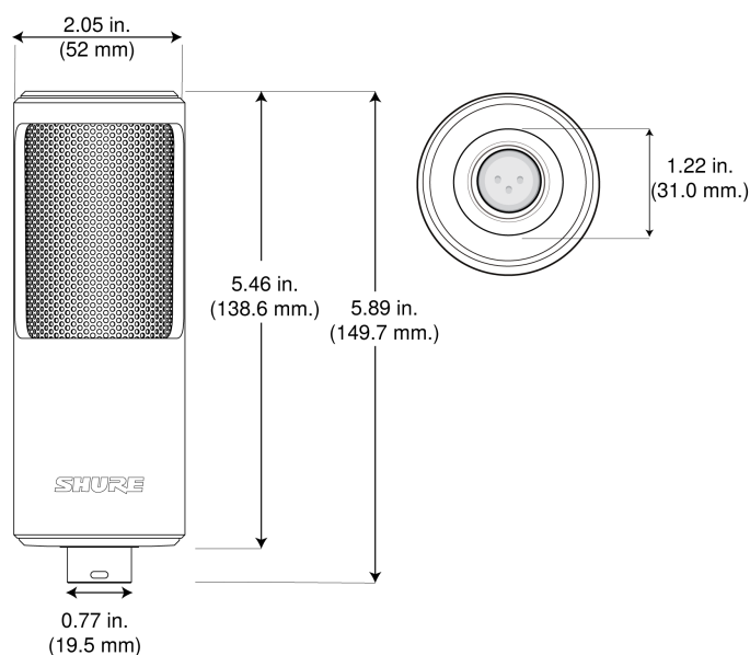
Dimensions du SM4
