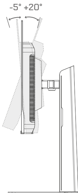
Inclinaison [-5° - +20°]
