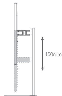
Réglage de la hauteur MBS27 : 150 mm MBS32 : 130 mm
