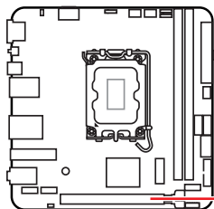
PCI_E1 : PCIe 5.0 x16 (depuis CPU)
